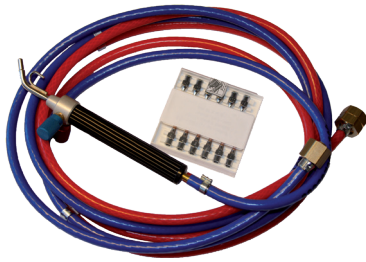
208797 Mikrobrenner loddepistol ink. sett med dyser.
